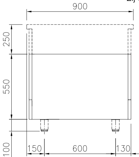
Zij aanzicht
